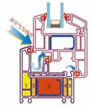
北新暖静门窗五腔室三密封结构图
